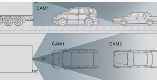
DBC 114066 TS / DBC 114047 TW Sichtfeld für Twin- und Tiltcameras Example for Viewing field of Twin- and Tiltcameras
